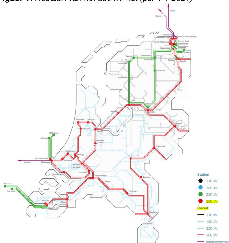
Figuur 1: Netkaart van het 380 kV-net (per 1-1-2021)
