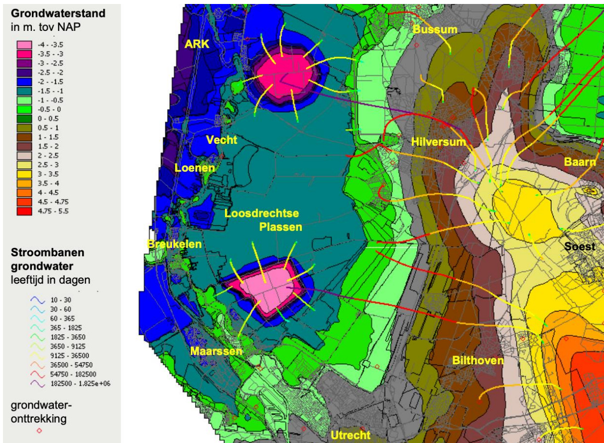
Figuur 5 Grondwaterstanden tussen het Gooi en de Vecht op basis van een geohydrologisch model. De grondwaterstroming verloopt loodrecht op de getoonde isohypsen, die punten met een gelijke stijghoogte (=grondwaterstand) met elkaar verbinden (Beemster, niet gepubl.)
